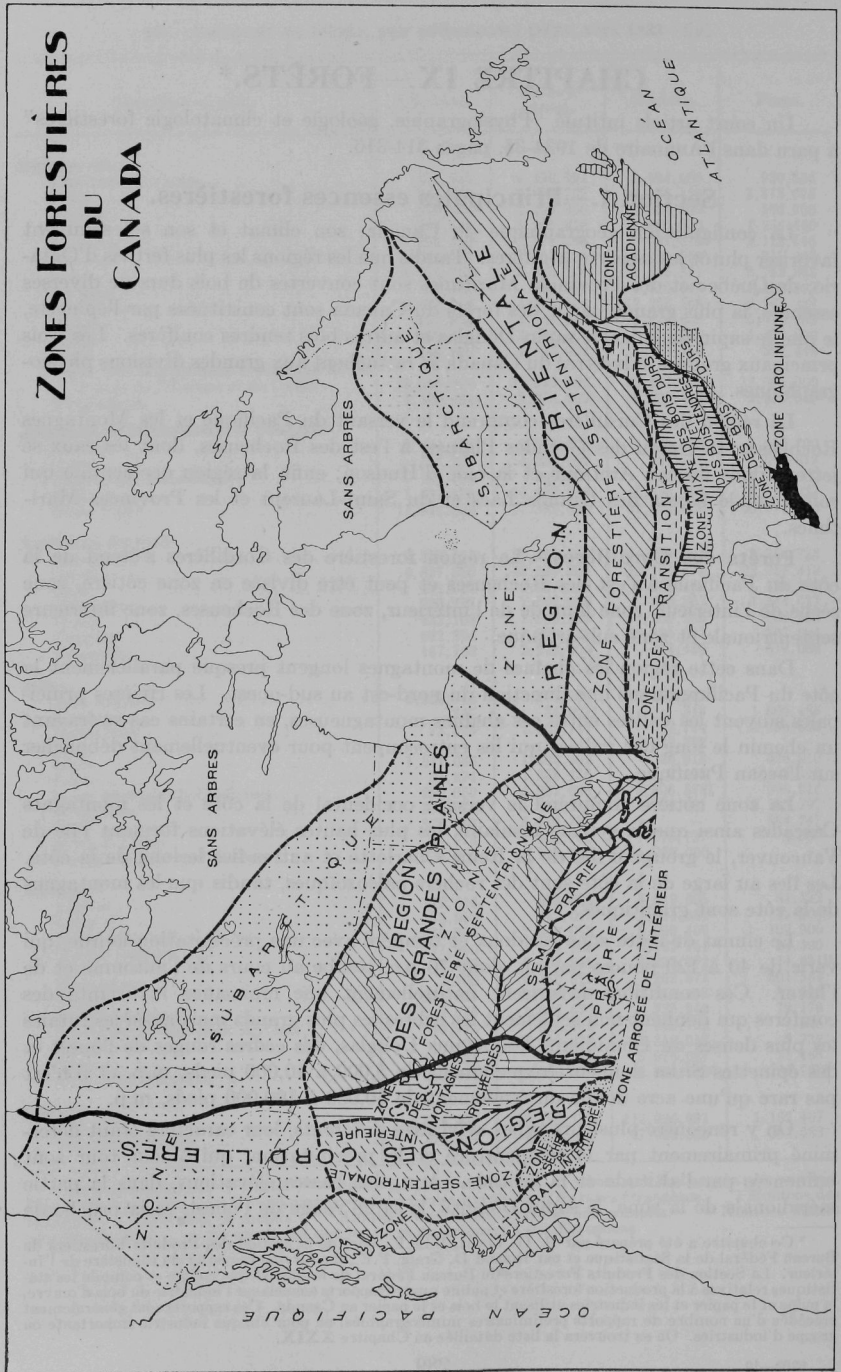
ZONES FORESTIÈRES DU CANADA.
